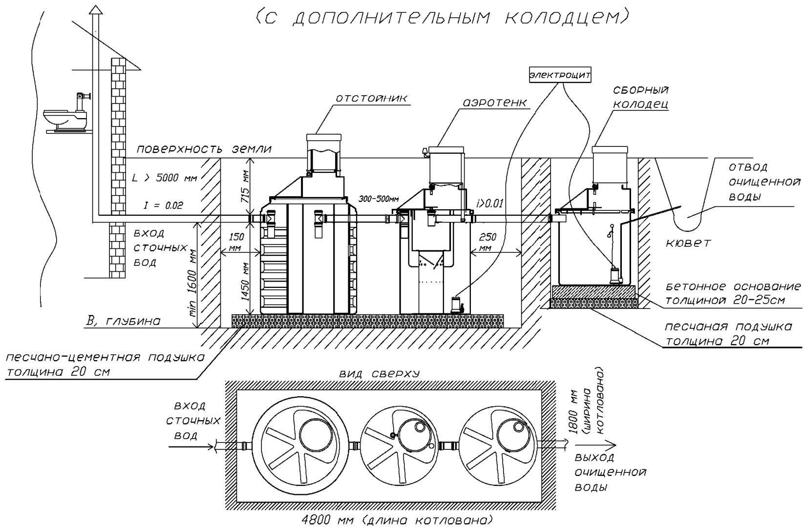
6.1. Монтажная схема ЛОС 5, 8 со сборным колодцем (песок, суглинок, глина)
