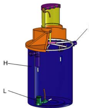
Рис. 4. Отстойник 1,5 м 3
