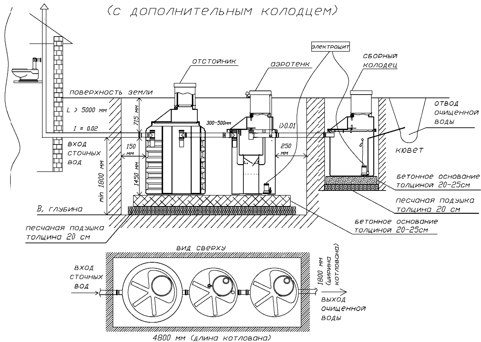
6.2. Монтажная схема ЛОС 5, 8 со сборным колодцем (пловун)
