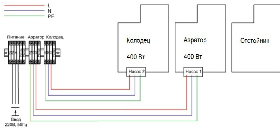
Рис. 9.1 Схема соединений установки ЛОС 8.
